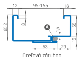
Oceľová zárubňa
